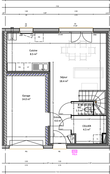
PLAN RDC
